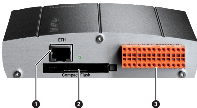
VideoJet X SN 系列 — 背面
